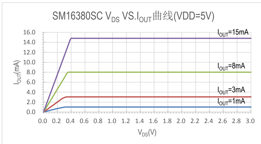
Fig. VDD=5V 时，SM16380SC I_{OUT} 与 V_{DS} 的关系曲线
