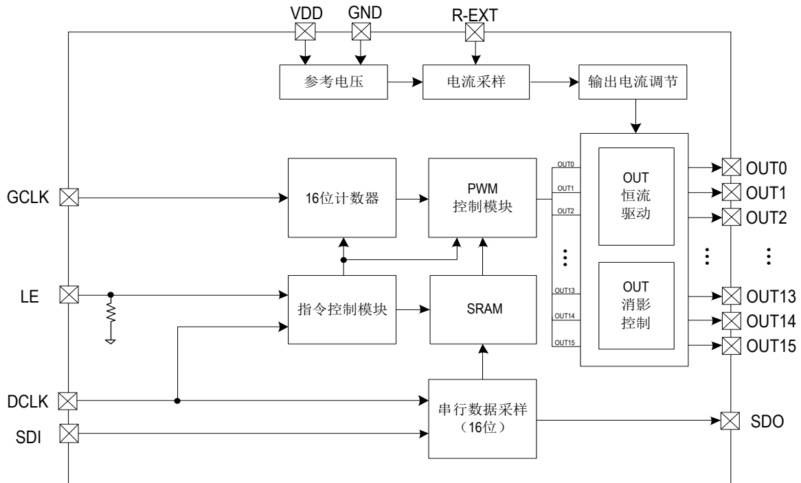
Fig. SM16380SC 内部功能框图
