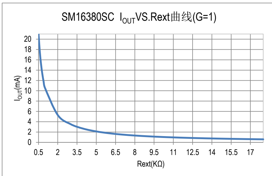
Fig. SM16380SC 的输出端口电流 I OUT 与 R EXT 电阻间的关系 (G=1)
